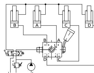
SCHEMA DI MONTAGGIO / ASSEMBLY GUIDE
